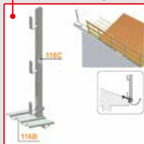
116 Parapetto sottotegola
