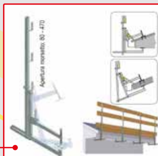
113B Parapetto inclinabile per calcestruzzo
