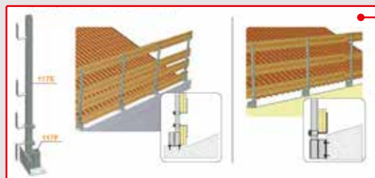
117G Parapetto per bordi orizzontali e verticali
