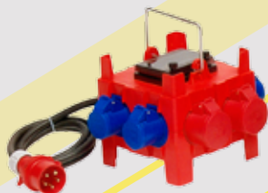
▼ QUADRI ELETTRICI PORTATILI PER CANTIERE
