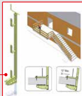
103 Parapetto universale con bascula
