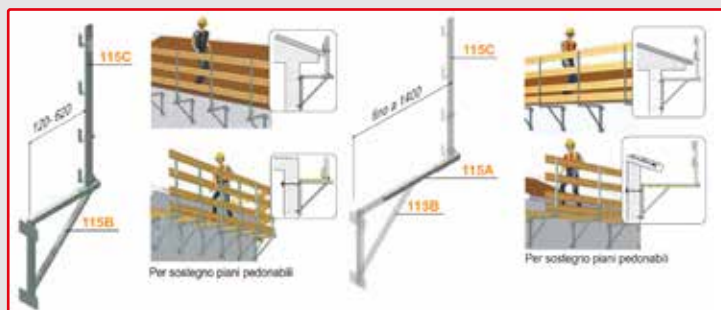
115BC Parapetto a mensola 12-62 + 115A prolunga per apertura fino a 140
